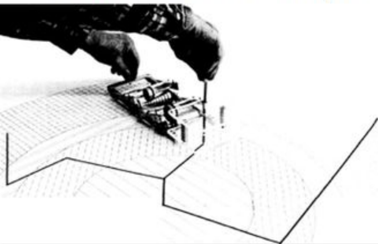
• FERMIAC
